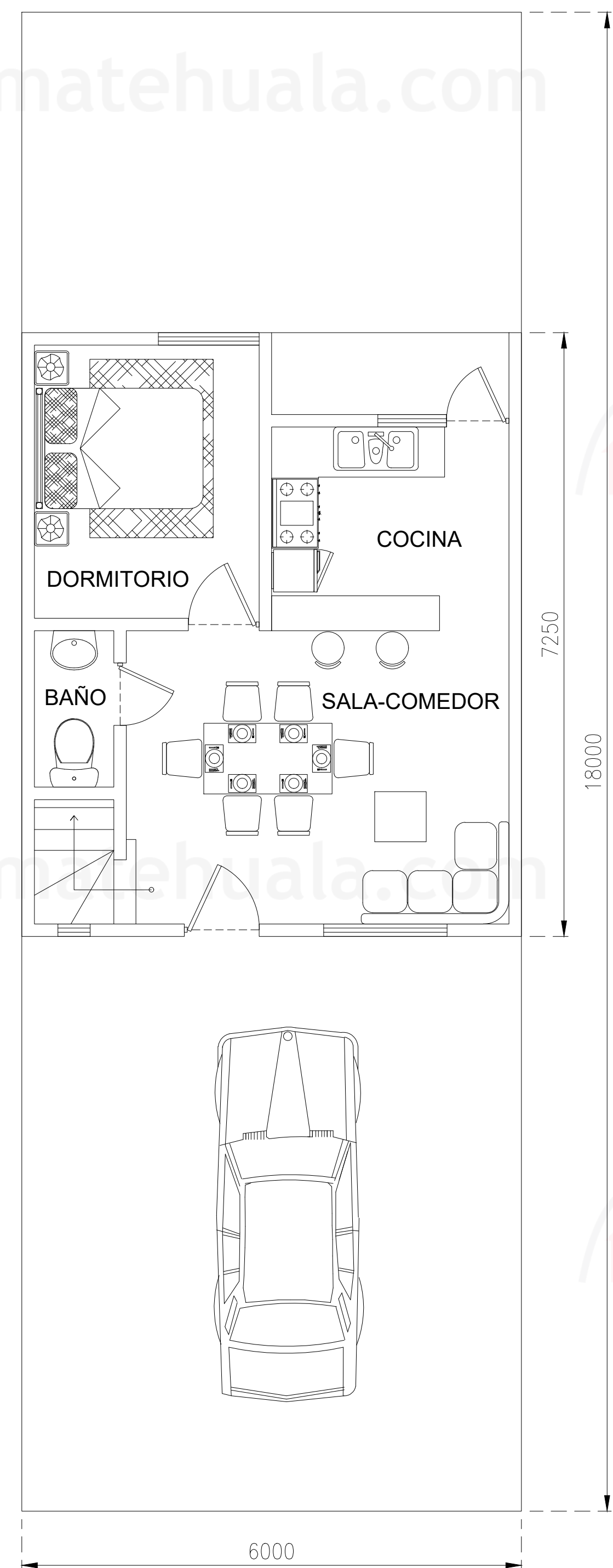
PROTOTIPO 3 COTAS EN CM SIN ESCALA
