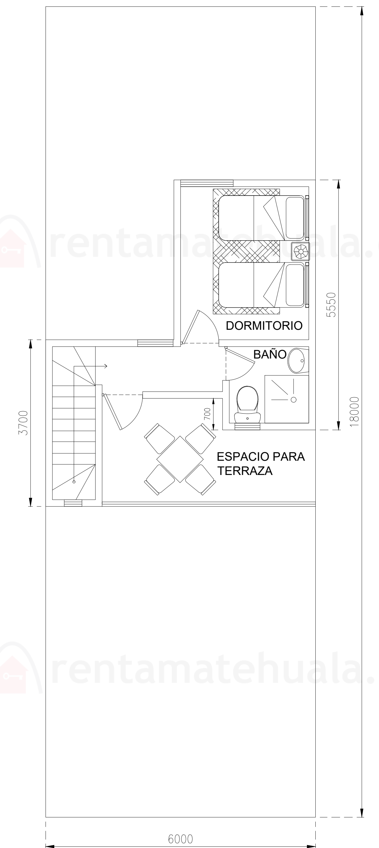
PROTOTIPO 3 COTAS EN CM SIN ESCALA
