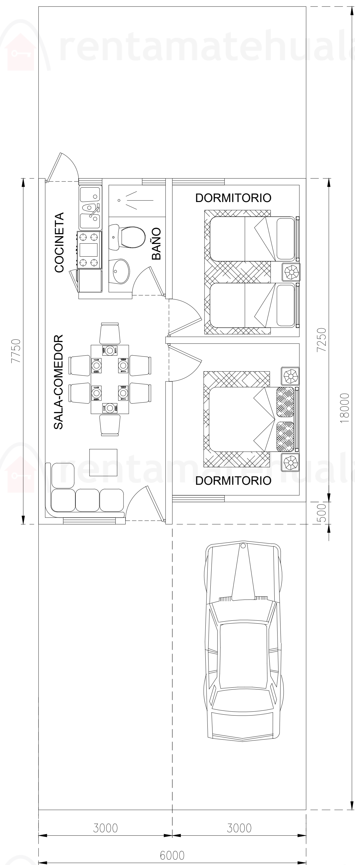
PROTOTIPO 1 COTAS EN CM SIN ESCALA
