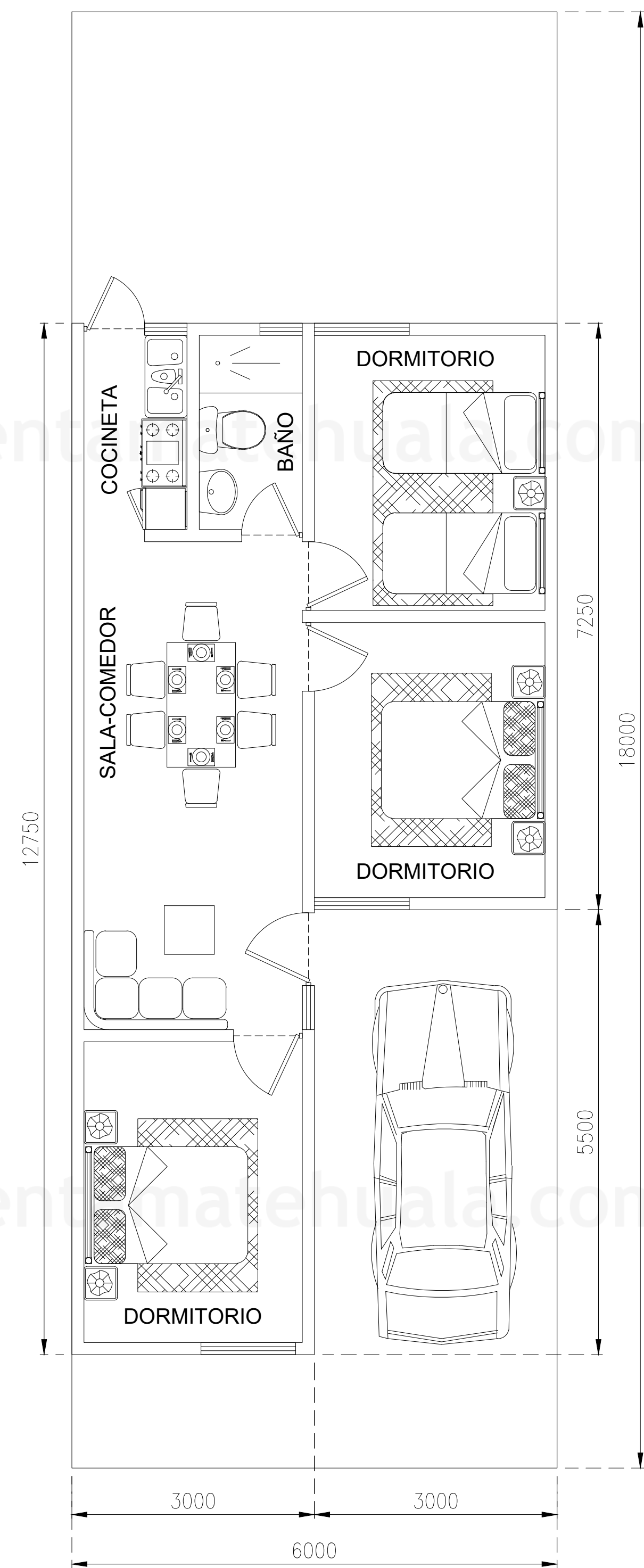
PROTOTIPO 2 COTAS EN CM SIN ESCALA
